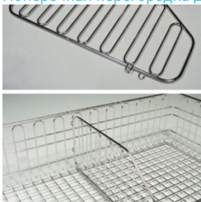
Поперечная перегородка для корзин со скосом 1/2 СтУ 282 x 141
